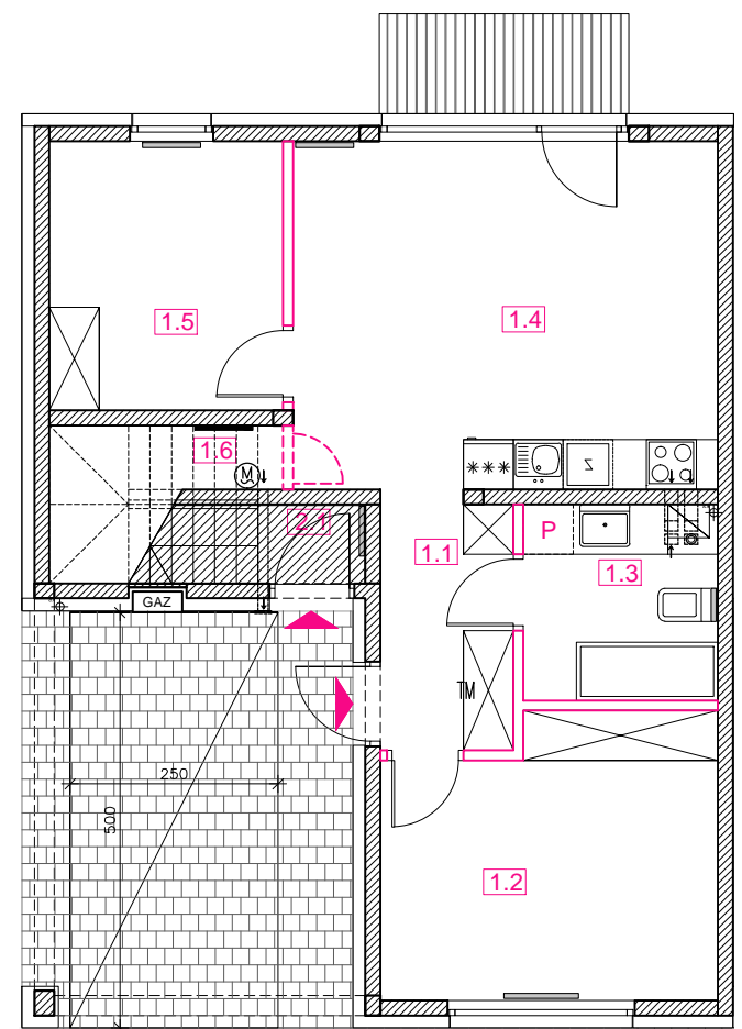
RZUT PARTERU
