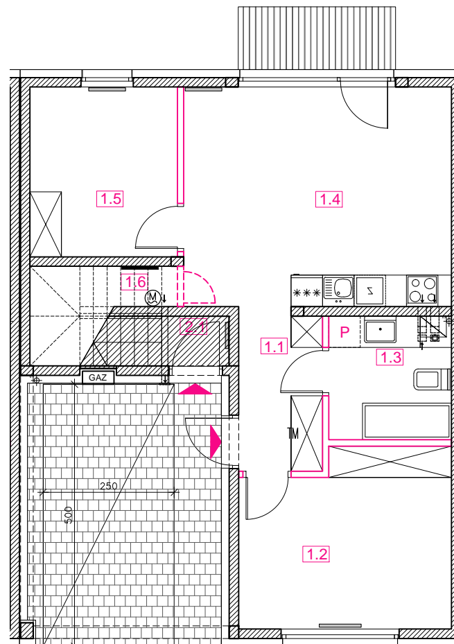
RZUT PARTERU
