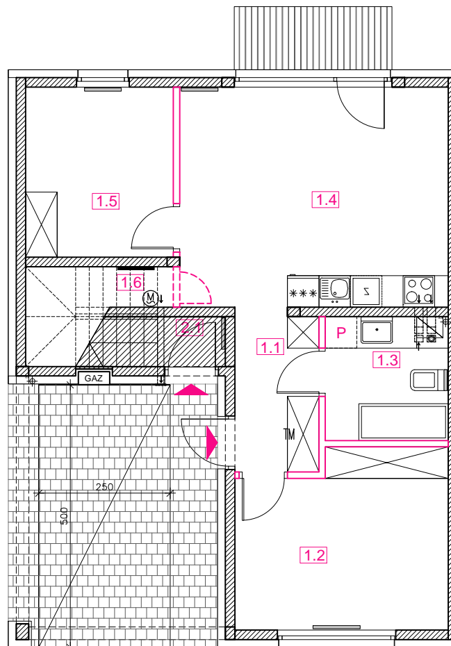
RZUT PARTERU
